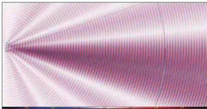
Simulacija NEODYMLINE 16 pri 4000Hz
