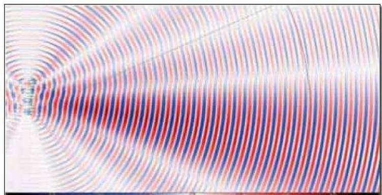
Simulacija NEODYMLINE 16 pri 800Hz
